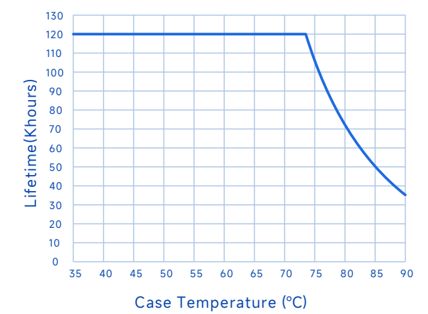
寿命Vs.壳温
