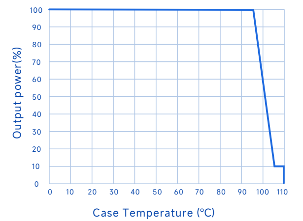
输出功率Vs.壳温
